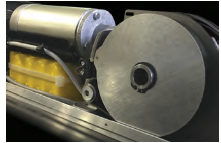
Batteries embarquées dans l'encombrement standard de l'automatisme.
