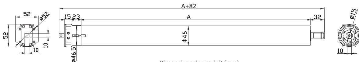
Dimensions du produit (mm)
